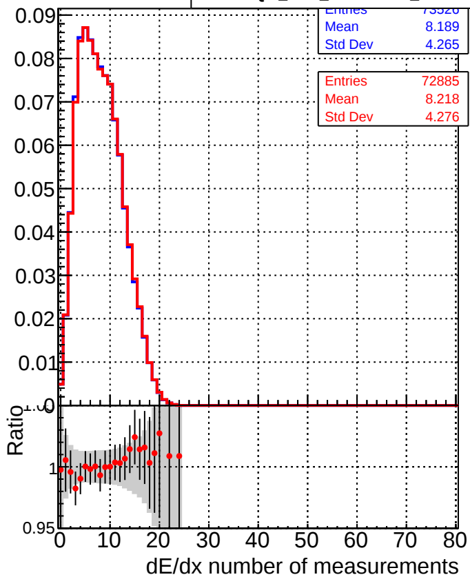
■ DQM_CKF_XiMinusPU_base ● DQM_CKF_XiMinusPU_retrainOldFiles125_v2_prelimWPM_epoch2
