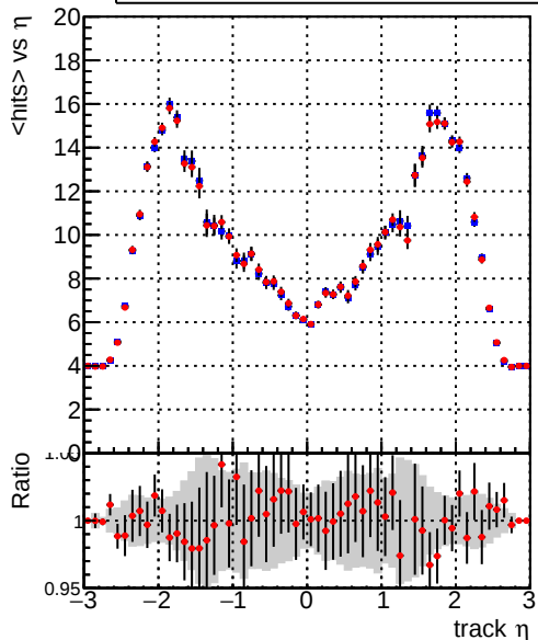
— DQM_CKF_XiMinusPU_base — DQM_CKF_XiMinusPU_retrainOldFiles125_v2_prelimWPM_epoch2
