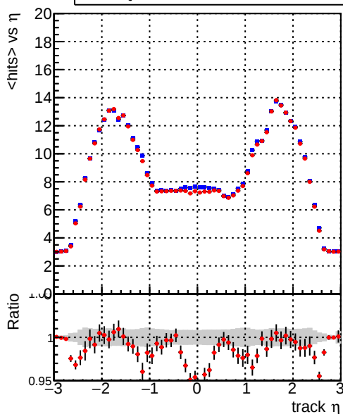
— DQM_CKF_XiMinusPU_base — DQM_CKF_XiMinusPU_retrainOldFiles125_v2_prelimWPM_epoch2
