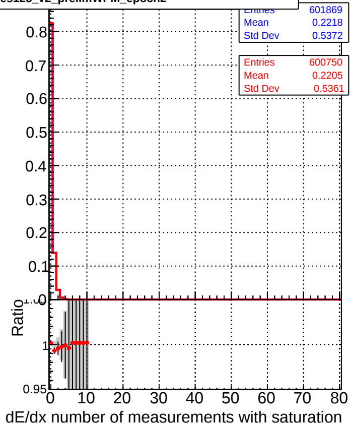
DQM_CKF_XiMinusPU_base DQM_CKF_XiMinusPU_retrainOldFiles125_v2_prelimWPM_epoch2
