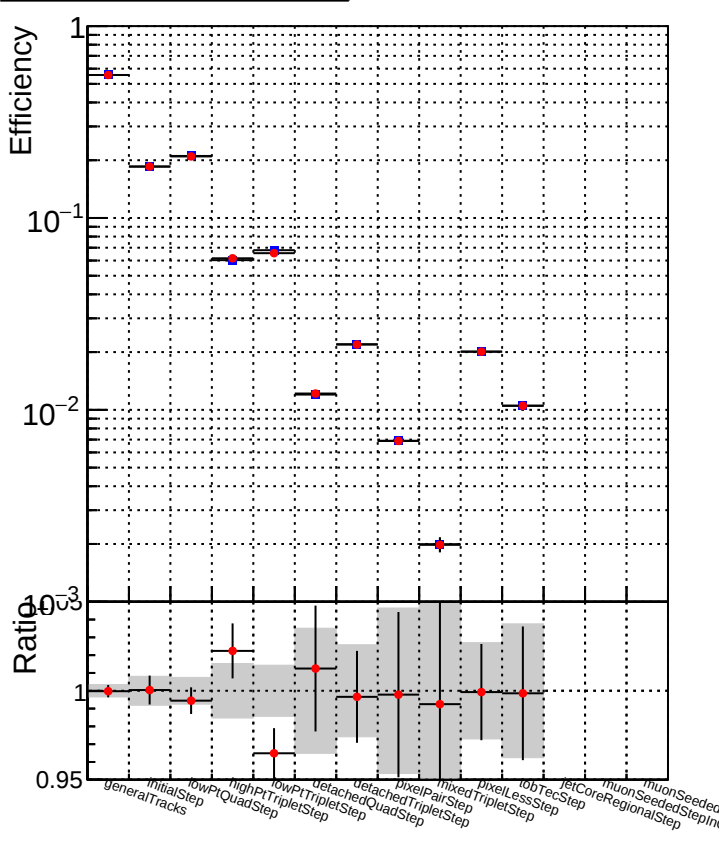
DQM_CKF_XiMinusPU_base DQM_CKF_XiMinusPU_retrainOldFiles125_v2_prelimWPM_epoch1
