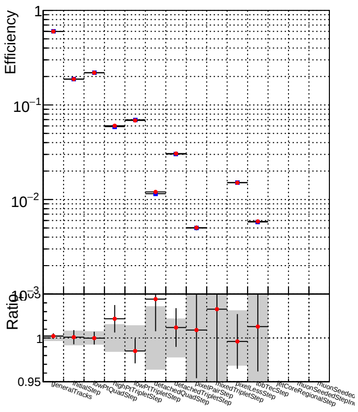
DQM_CKF_XiMinusPU_base DQM_CKF_XiMinusPU_retrainOldFiles125_v2_prelimWPM_epoch1
