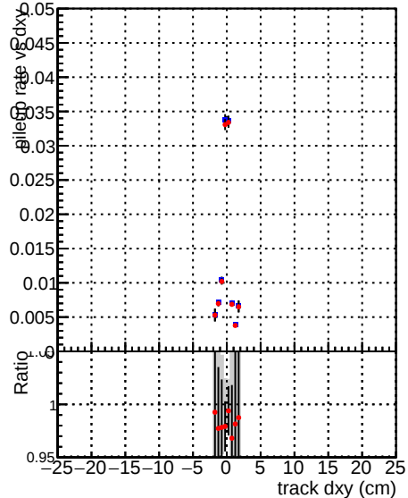
DQM CKF_XiMinusPU_retrainOldFiles125_v2_prelimWPM_epoch1
