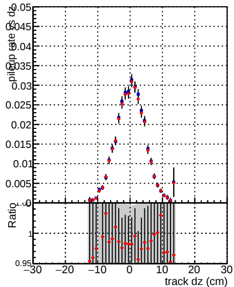
DQM CKF_XiMinusPU_retrainOldFiles125_v2_prelimWPM_epoch1
