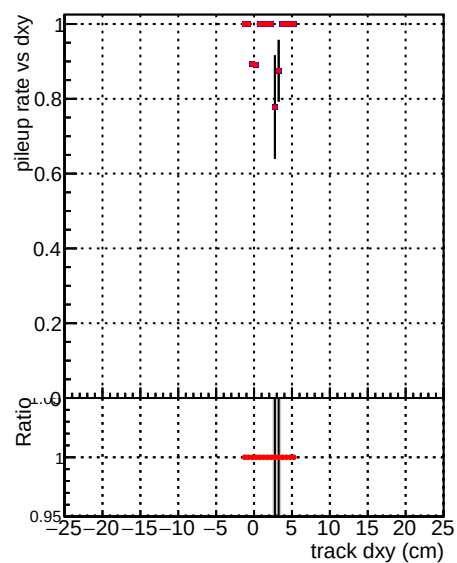
DQM CKF_XiMinusPU_retrainOldFiles125_v2_prelimWPM_epoch1
