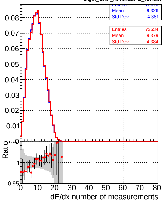
DQM_CKF_XiMinusPU_base DQM_CKF_XiMinusPU_retrainOldFiles125_v2_prelimWPM_epoch1
