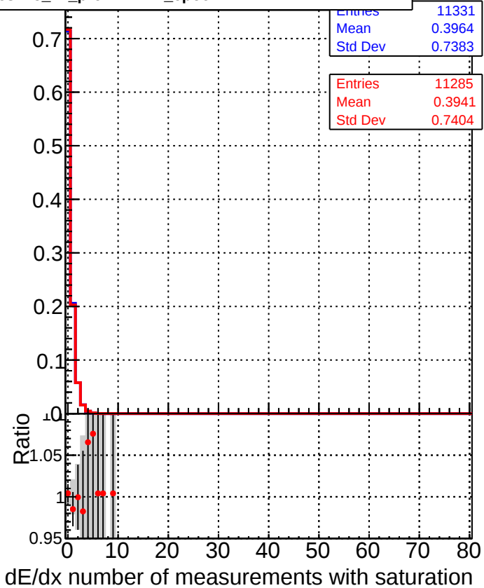
■ DQM_CKF_XiMinusPU_base ● DQM_CKF_XiMinusPU_retrainOldFiles125_v2_prelimWPM_epoch1
