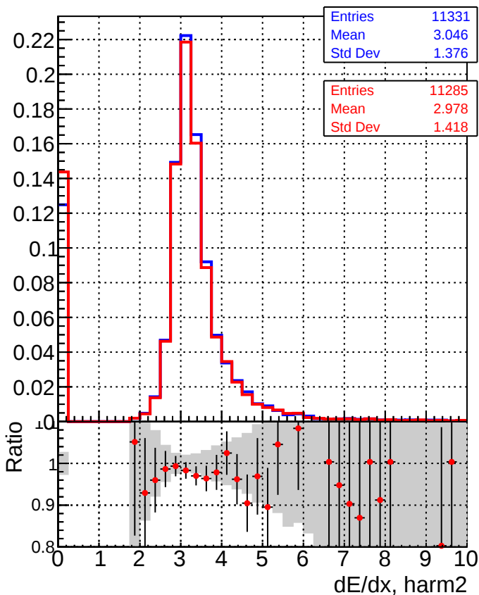
■ DQM_CKF_XiMinusPU_base ● DQM_CKF_XiMinusPU_retrainOldFiles125_v2_prelimWPM_epoch1
