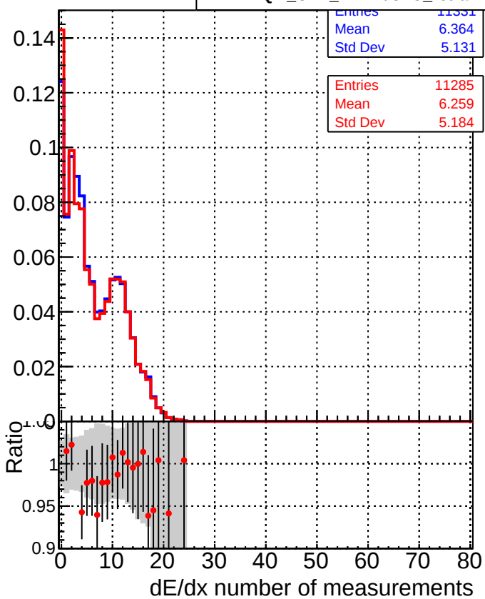
■ DQM_CKF_XiMinusPU_base ● DQM_CKF_XiMinusPU_retrainOldFiles125_v2_prelimWPM_epoch1
