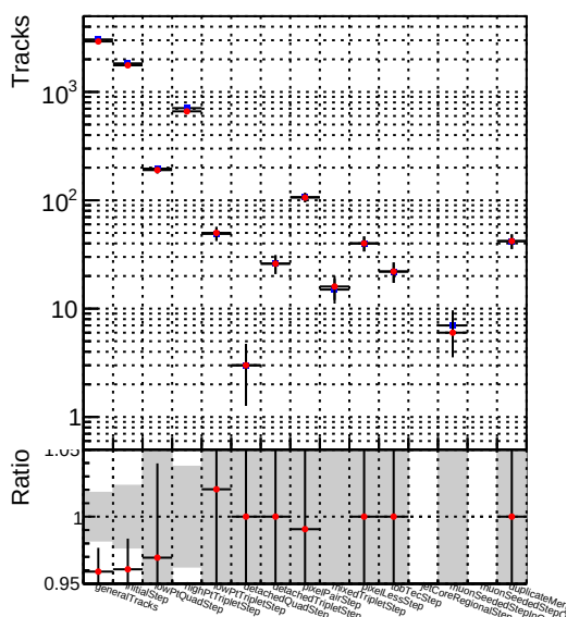
—■ DQM_CKF_XiMinusPU_base
