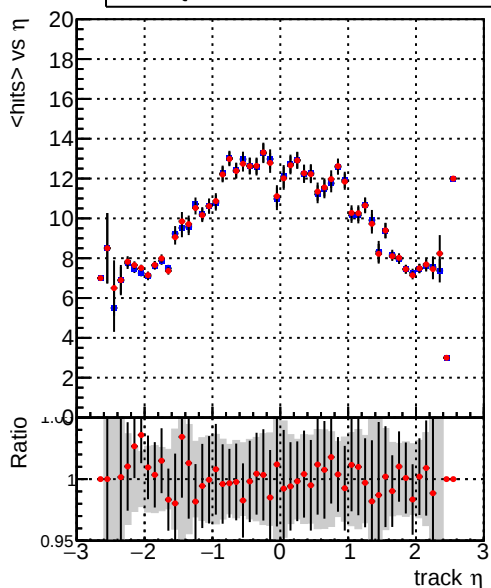
— DQM_CKF_XiMinusPU_base — DQM_CKF_XiMinusPU_retrainOldFiles125_v2_prelimWPM_epoch1
