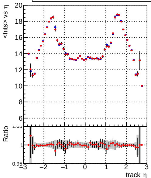
— DQM_CKF_XiMinusPU_base — DQM_CKF_XiMinusPU_retrainOldFiles125_v2_prelimWPM_epoch1
