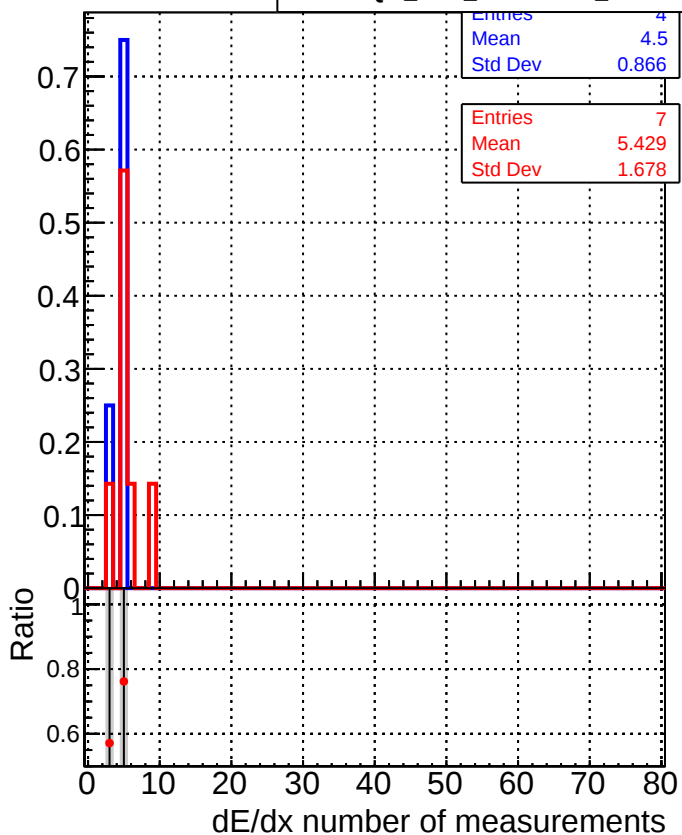
■ DQM_CKF_XiMinusPU_base ■ DQM_CKF_XiMinusPU_retrainOldFiles125_v2_prelimWPM_epoch1
