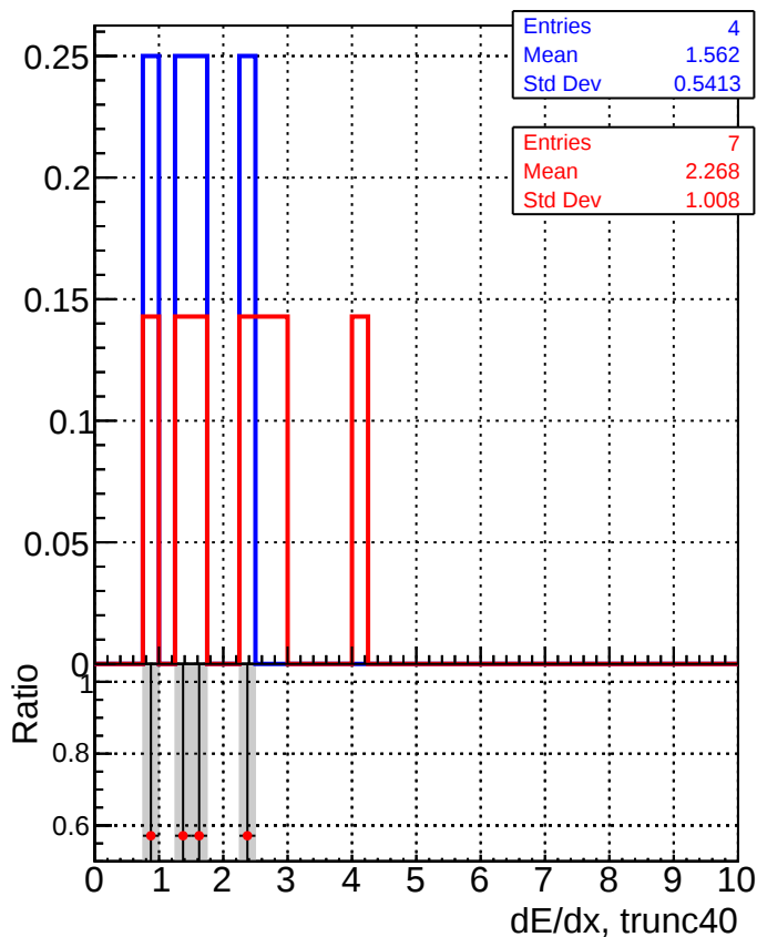
■ DQM_CKF_XiMinusPU_base ■ DQM_CKF_XiMinusPU_retrainOldFiles125_v2_prelimWPM_epoch1
