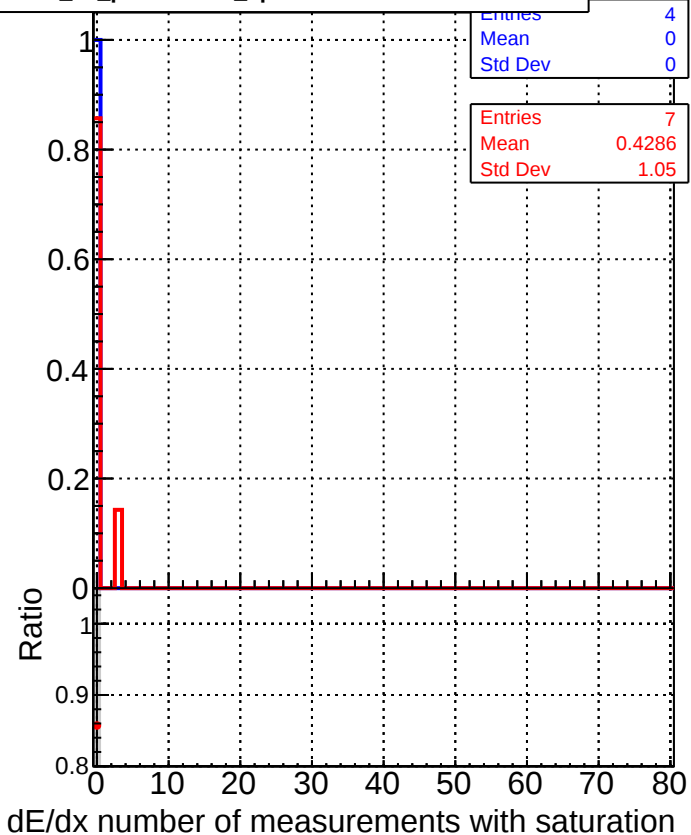
■ DQM_CKF_XiMinusPU_base ■ DQM_CKF_XiMinusPU_retrainOldFiles125_v2_prelimWPM_epoch1
