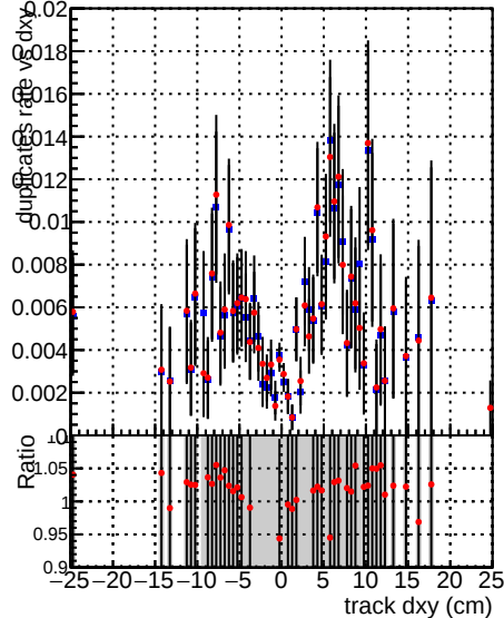
—◆— DQM_CKF_XiMinusPU_base —●— DQM_CKF_XiMinusPU_retrainOldFiles125_v2_prelimWPM_epoch1
