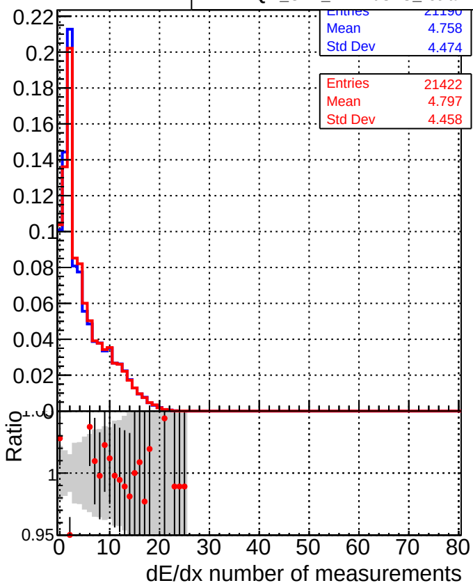
■ DQM_CKF_XiMinusPU_base ● DQM_CKF_XiMinusPU_retrainOldFiles125_v2_prelimWPM_epoch1
