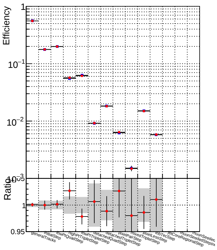
DQM_CKF_XiMinusPU_base DQM_CKF_XiMinusPU_retrainOldFiles125_v2_prelimWPM_epoch0
