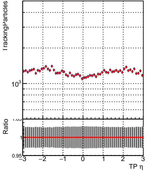
■ DQM_CKF_XiMinusPU_base ■ DQM_CKF_XiMinusPU_retrainOldFiles125_v2_prelimWPM_epoch0
