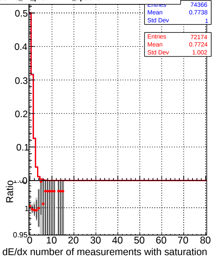
DQM_CKF_XiMinusPU_base DQM_CKF_XiMinusPU_retrainOldFiles125_v2_prelimWPM_epoch0
