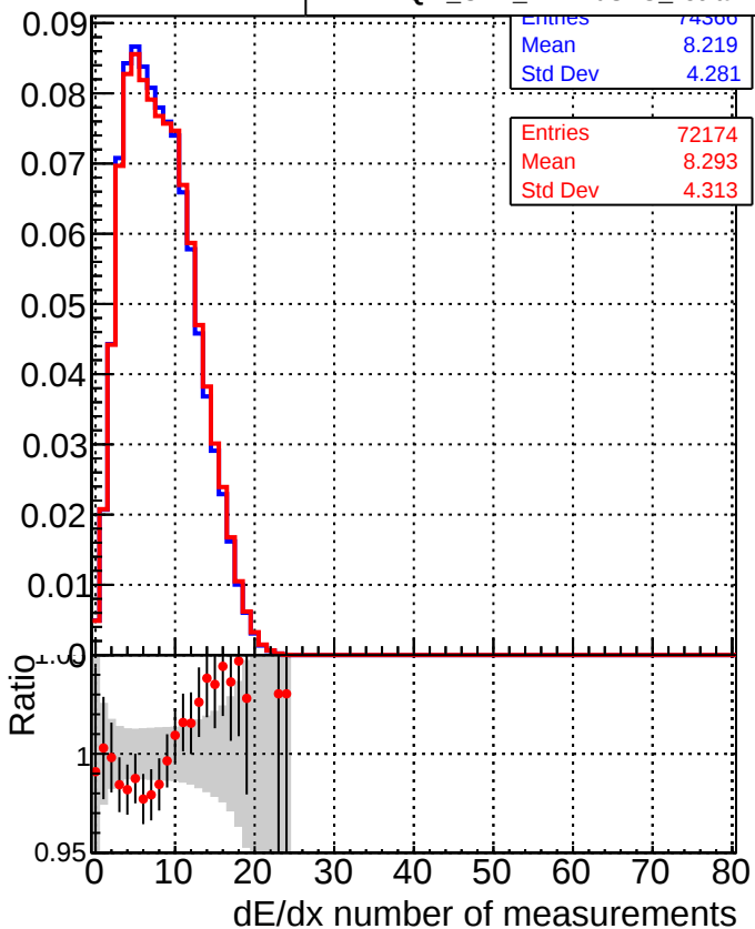
DQM_CKF_XiMinusPU_base DQM_CKF_XiMinusPU_retrainOldFiles125_v2_prelimWPM_epoch0
