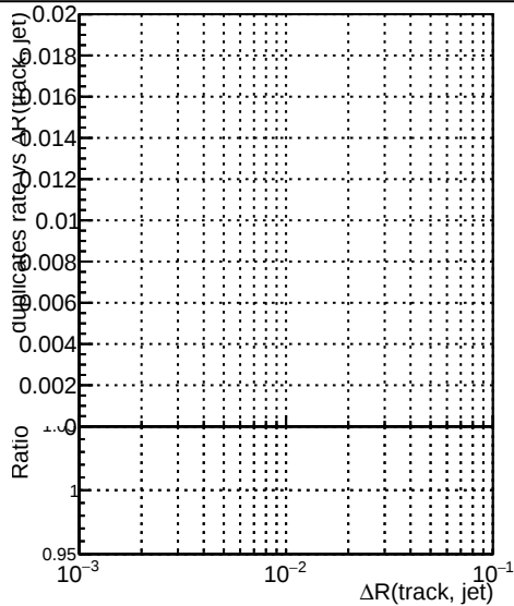
—•— DQM_CKF_XiMinusPU_base —•— DQM_CKF_XiMinusPU_retrainOldFiles125_v2_prelimWPM_epoch0
