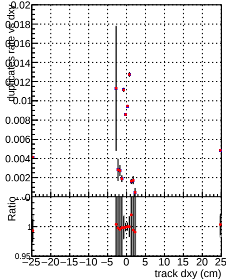
DQM CKF_XiMinusPU_base
