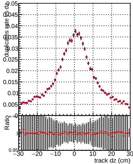
DQM CKF_XiMinusPU_base
