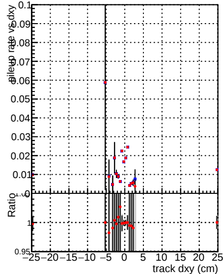
DQM CKF_XiMinusPU_retrainOldFiles125_v2_prelimWPM_epoch0
