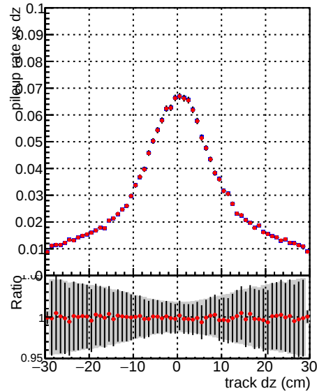
DQM CKF_XiMinusPU_retrainOldFiles125_v2_prelimWPM_epoch0
