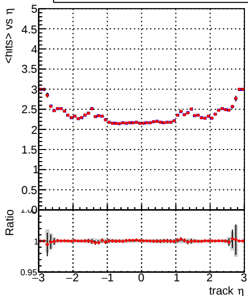
mean hits — DQM_CKF_XiMinusPU_base — DQM_CKF_XiMinusPU_retrainOldFiles125_v2_prelimWPM_epoch0
