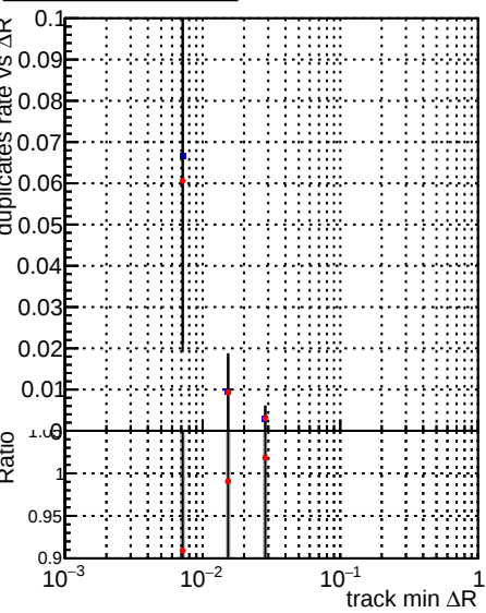
—•— DQM_CKF_XiMinusPU_base —•— DQM_CKF_XiMinusPU_retrainOldFiles125_v2_prelimWPM_epoch0
