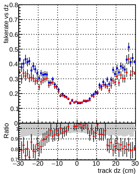
—●— DQM CKF_XiMinusPU_base —●— DQM CKF_XiMinusPU_retrainOldFiles125_v2_prelimWPM_epoch0
