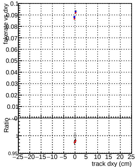
—●— DQM_CKF_XiMinusPU_base —●— DQM_CKF_XiMinusPU_retrainOldFiles125_v2_prelimWPM_epoch0
