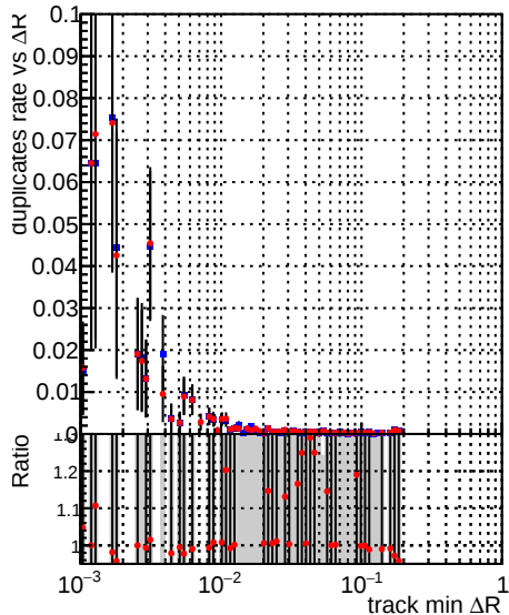
—●— DQM_CKF_XiMinusPU_base —●— DQM_CKF_XiMinusPU_retrainOldFiles125_v2_prelimWPM_epoch0
