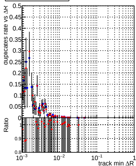
—•— DQM_CKF_XiMinusPU_base —•— DQM_CKF_XiMinusPU_retrainOldFiles125_v2_prelimWPM_epoch0
