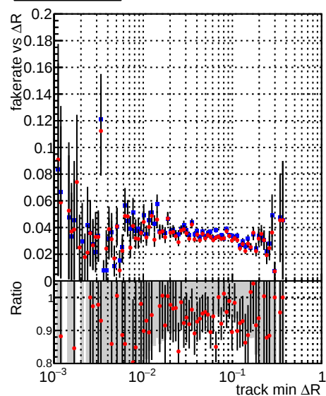
—•— DQM_CKF_XiMinusPU_base —•— DQM_CKF_XiMinusPU_retrainOldFiles125_v2_prelimWPM_epoch0
