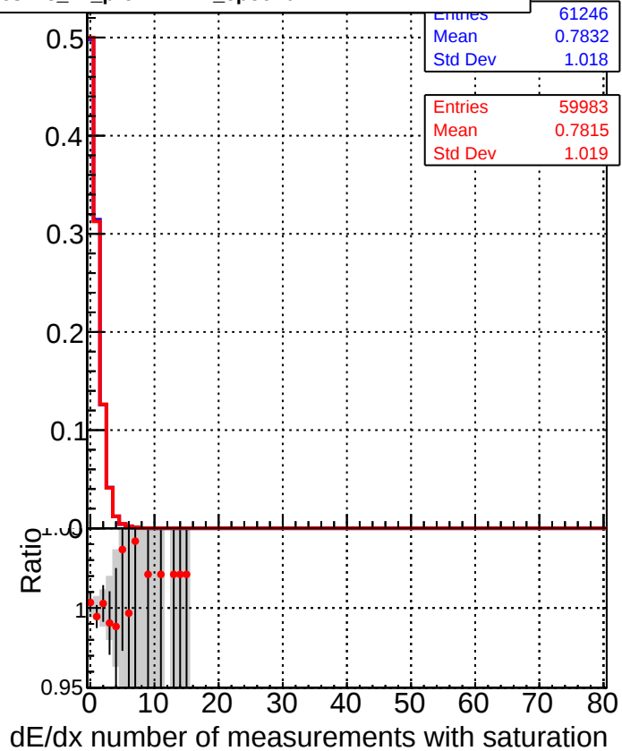
DQM_CKF_XiMinusPU_base DQM_CKF_XiMinusPU_retrainOldFiles125_v2_prelimWPM_epoch0
