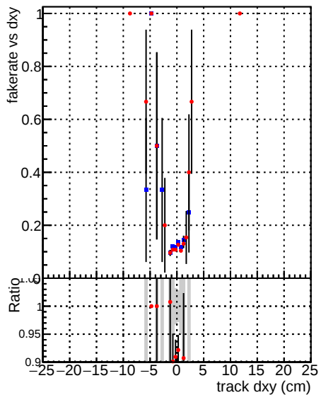
—●— DQM_CKF_XiMinusPU_base —●— DQM_CKF_XiMinusPU_retrainOldFiles125_v2_prelimWPM_epoch0
