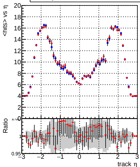
mean hits — DQM_CKF_XiMinusPU_base — DQM_CKF_XiMinusPU_retrainOldFiles125_v2_prelimWPM_epoch0
