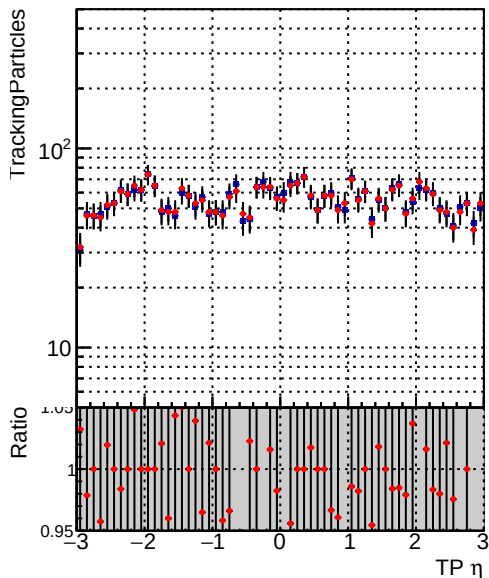
—●— DQM_CKF_XiMinusPU_base —●— DQM_CKF_XiMinusPU_retrainOldFiles125_v2_prelimWPM_epoch0
