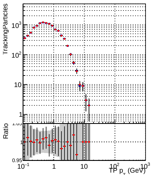
—●— DQM_CKF_XiMinusPU_base —●— DQM_CKF_XiMinusPU_retrainOldFiles125_v2_prelimWPM_epoch0
