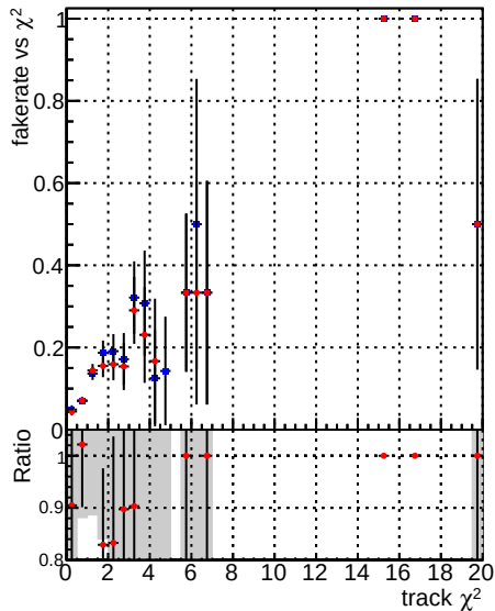
Fake rate vs. \chi^2 —●— DQM CKF XiMinusPU base —●— DQM CKF XiMinusPU_retrainOldFiles125_v2_prelimWPM_epoch0
