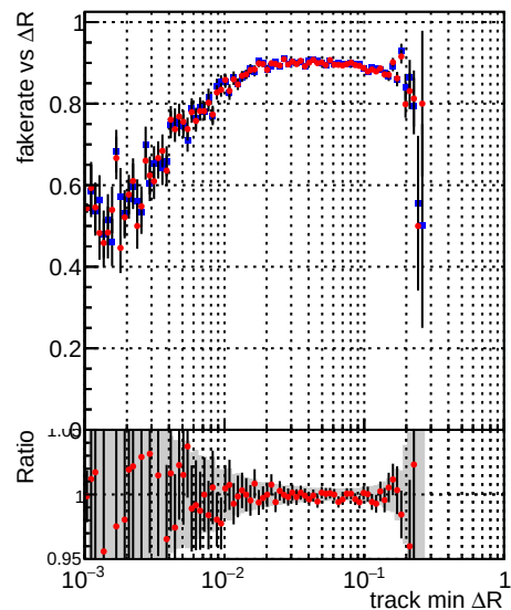
—•— DQM_CKF_XiMinusPU_base —•— DQM_CKF_XiMinusPU_retrainOldFiles125_v2_prelimWPM_epoch0
