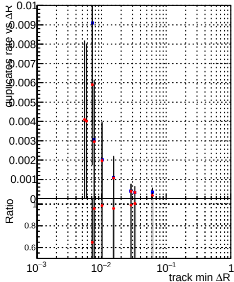
—•— DQM_CKF_XiMinusPU_base —•— DQM_CKF_XiMinusPU_retrainOldFiles125_v2_prelimWPM_epoch0
