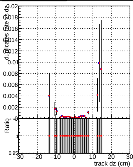
— DQM_CKF_XiMinusPU_base — DQM_CKF_XiMinusPU_retrainOldFiles125_v2_prelimWPM_epoch0
