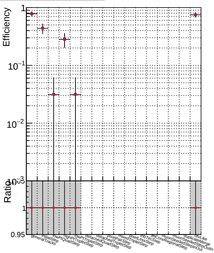
DQM_CKF_XiMinusPU_base DQM_CKF_XiMinusPU_retrainOldFiles125_v2_prelimWPM_epoch0
