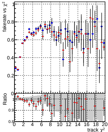
Fake rate vs. —◆— DQM CKF XiMinusPU_base —★— DQM CKF XiMinusPU_retrainOldFiles125_v2_prelimWPM_epoch0
