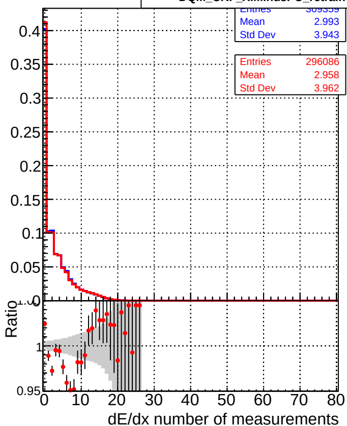
■ DQM_CKF_XiMinusPU_base ● DQM_CKF_XiMinusPU_retrainOldFiles125_v2_prelimWPM_epoch0
