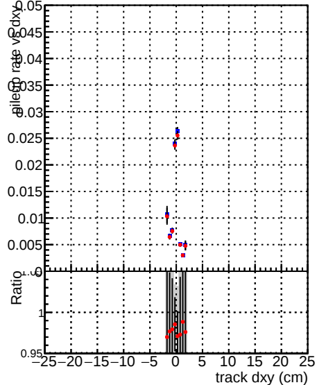
DQM CKF_XiMinusNOPU_retrainOldFiles125_v2_prelimWPM_epoch4
