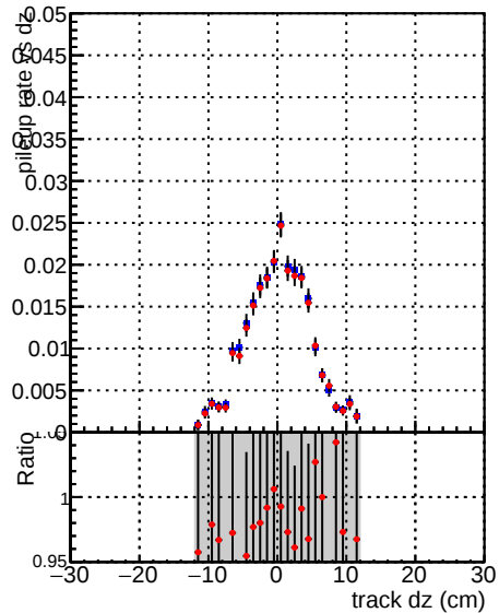
DQM CKF_XiMinusNOPU_retrainOldFiles125_v2_prelimWPM_epoch4
