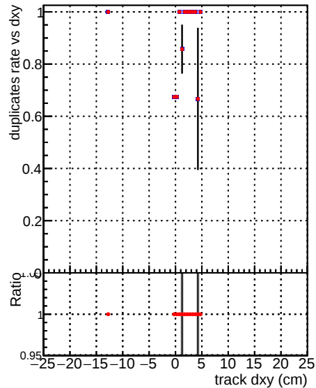
—●— DQM_CKF_XiMinusNOPU_base —●— DQM_CKF_XiMinusNOPU_retrainOldFiles125_v2_prelimWPM_epoch4
