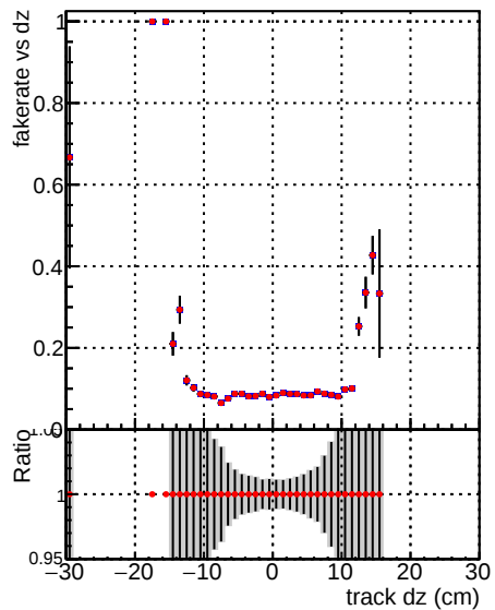
—●— DQM_CKF_XiMinusNOPU_base —●— DQM_CKF_XiMinusNOPU_retrainOldFiles125_v2_prelimWPM_epoch4
