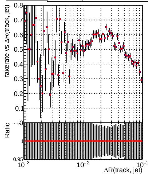
—●— DQM_CKF_XiMinusNOPU_base —●— DQM_CKF_XiMinusNOPU_retrainOldFiles125_v2_prelimWPM_epoch4
