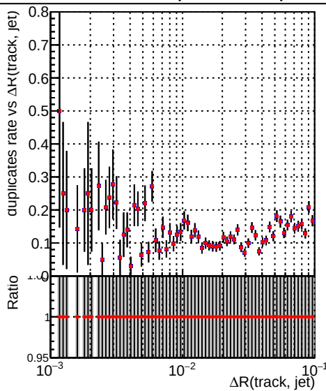
—●— DQM_CKF_XiMinusNOPU_base —●— DQM_CKF_XiMinusNOPU_retrainOldFiles125_v2_prelimWPM_epoch4
