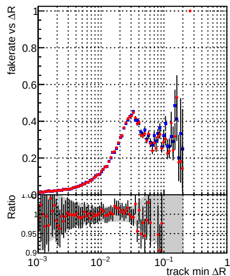
—●— DQM_CKF_XiMinusNOPU_base —●— DQM_CKF_XiMinusNOPU_retrainOldFiles125_v2_prelimWPM_epoch4
