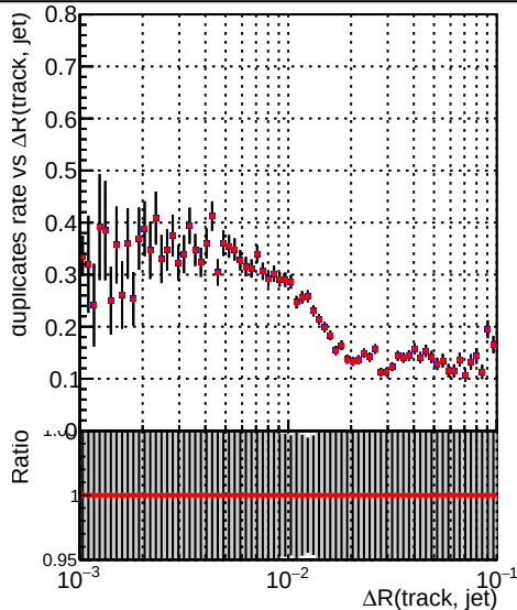
—•— DQM_CKF_XiMinusNOPU_base —•— DQM_CKF_XiMinusNOPU_retrainOldFiles125_v2_prelimWPM_epoch4
