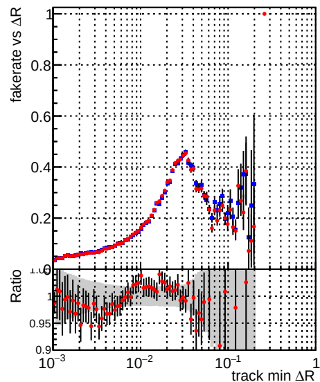
—•— DQM_CKF_XiMinusNOPU_base —•— DQM_CKF_XiMinusNOPU_retrainOldFiles125_v2_prelimWPM_epoch4
