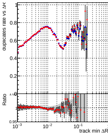
—•— DQM_CKF_XiMinusNOPU_base —•— DQM_CKF_XiMinusNOPU_retrainOldFiles125_v2_prelimWPM_epoch4
