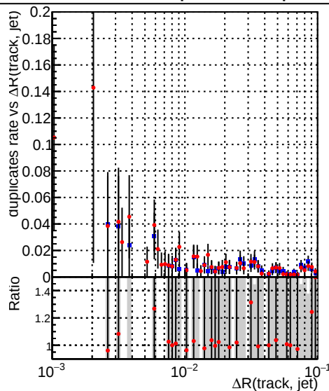
—•— DQM_CKF_XiMinusNOPU_base —•— DQM_CKF_XiMinusNOPU_retrainOldFiles125_v2_prelimWPM_epoch4
