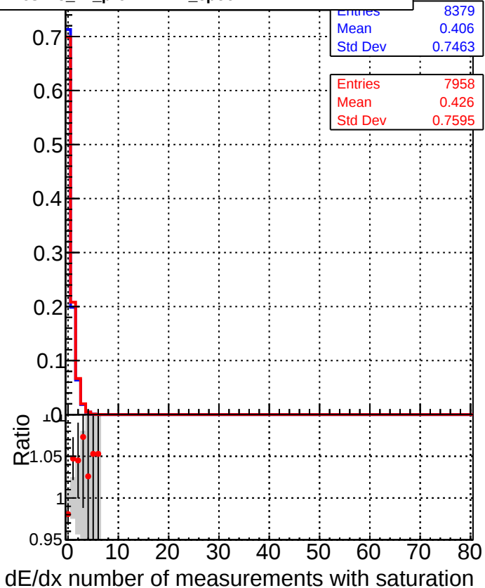
■ DQM_CKF_XiMinusNOPU_base ● DQM_CKF_XiMinusNOPU_retrainOldFiles125_v2_prelimWPM_epoch4
