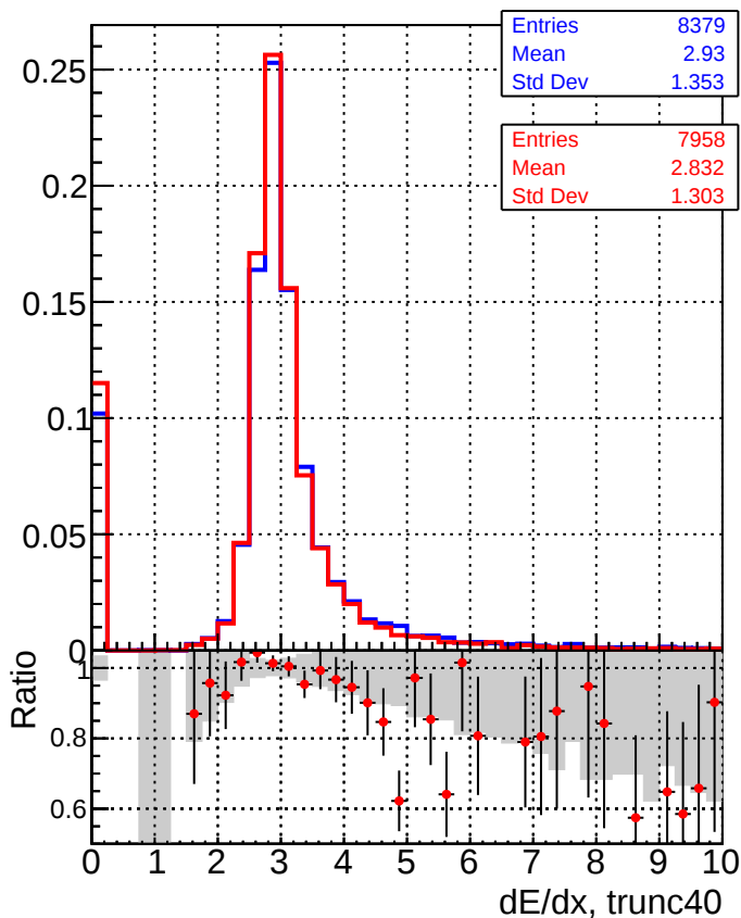
■ DQM_CKF_XiMinusNOPU_base ● DQM_CKF_XiMinusNOPU_retrainOldFiles125_v2_prelimWPM_epoch4
