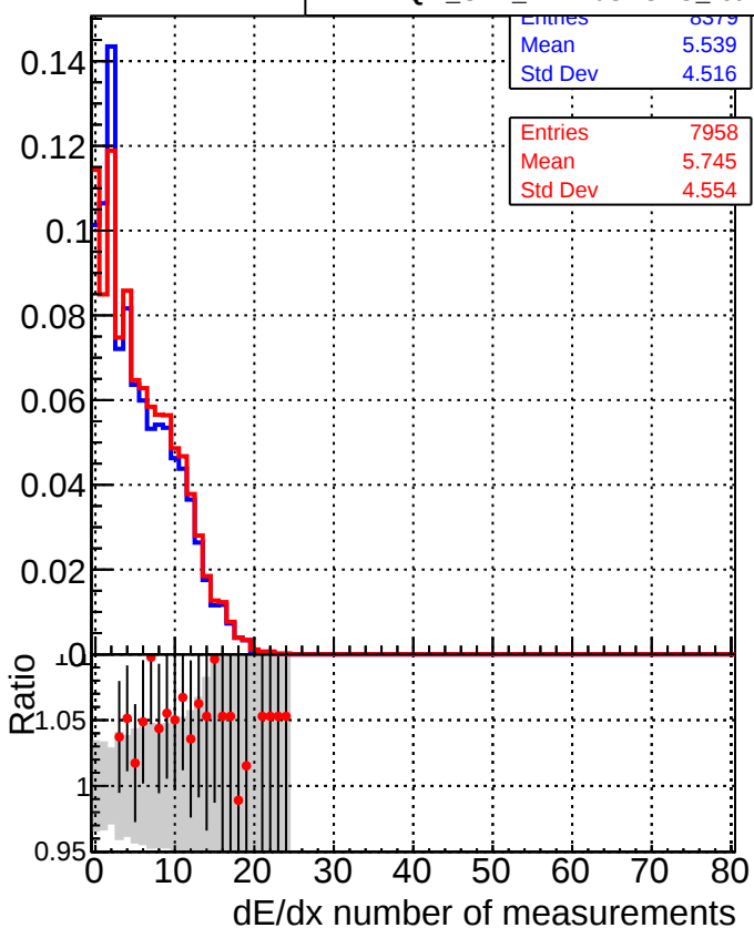
■ DQM_CKF_XiMinusNOPU_base ● DQM_CKF_XiMinusNOPU_retrainOldFiles125_v2_prelimWPM_epoch4
