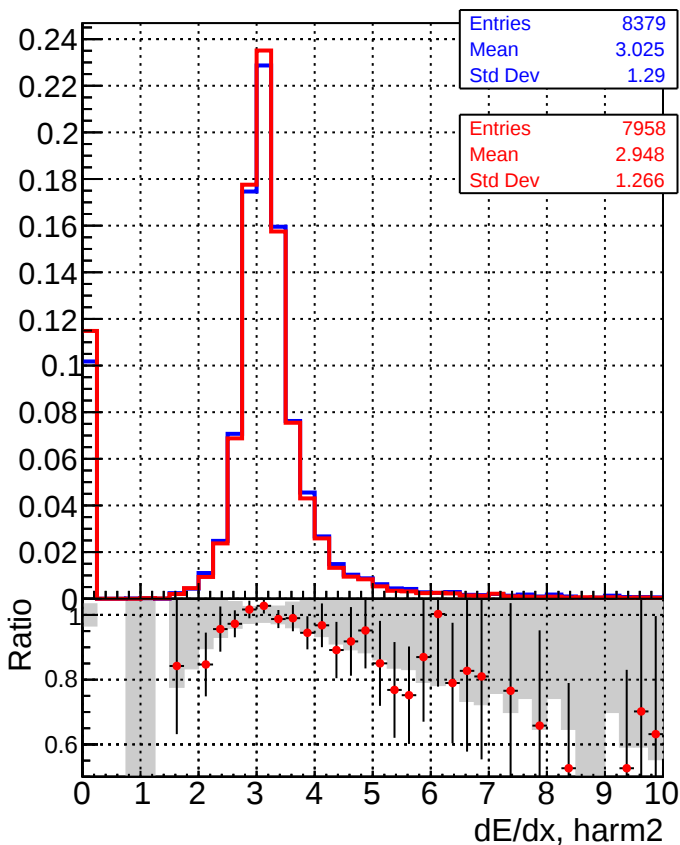
■ DQM_CKF_XiMinusNOPU_base ● DQM_CKF_XiMinusNOPU_retrainOldFiles125_v2_prelimWPM_epoch4
