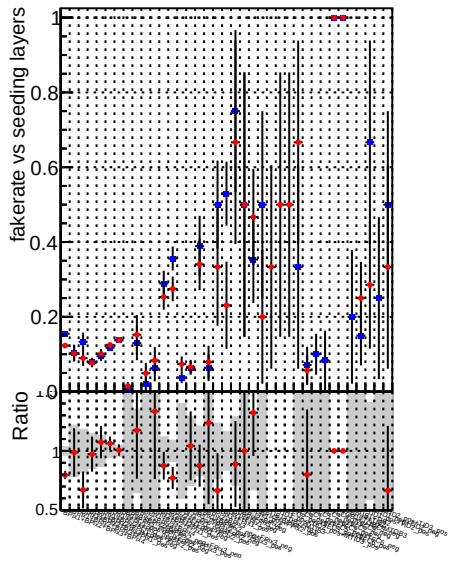
Fake rate vs. —◆— DQM CKF XiMinusNOPU_base —◆— DQM CKF XiMinusNOPU_retrainOldFiles125_v2_prelimWPM_epoch4
