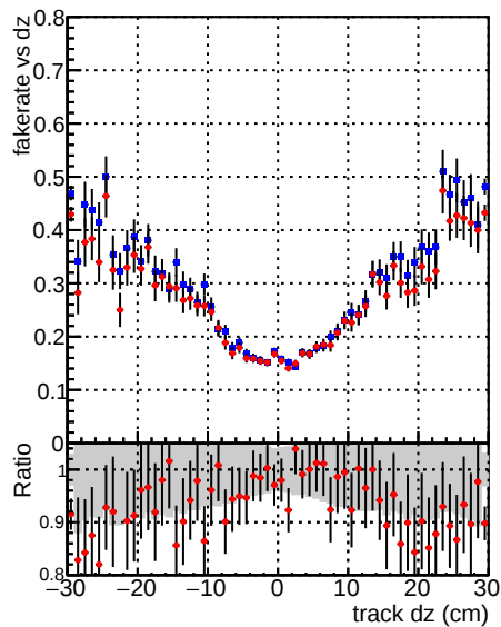
—●— DQM CKF XiMinusNOPU_base —●— DQM CKF XiMinusNOPU_retrainOldFiles125_v2_prelimWPM_epoch4
