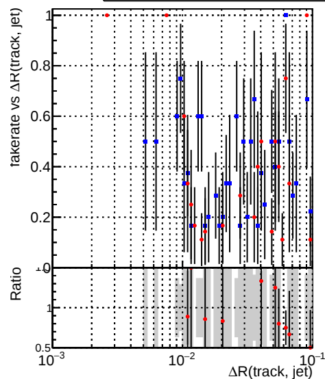
—•— DQM_CKF_XiMinusNOPU_base —•— DQM_CKF_XiMinusNOPU_retrainOldFiles125_v2_prelimWPM_epoch4
