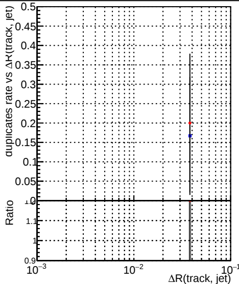
—•— DQM_CKF_XiMinusNOPU_base —•— DQM_CKF_XiMinusNOPU_retrainOldFiles125_v2_prelimWPM_epoch4
