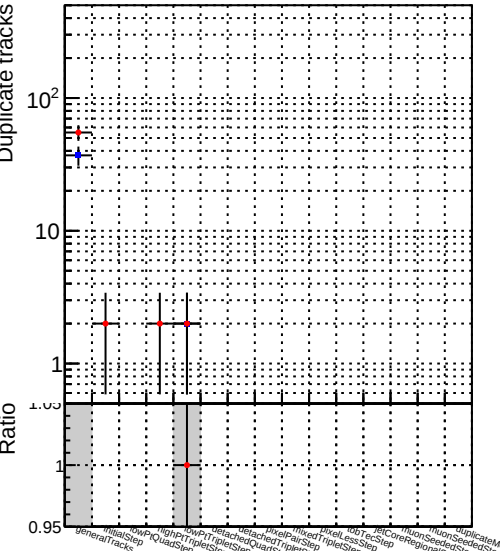
Numbe —●— DQM_CKF XiMinusNOPU retrainOldFiles125 v2 prelimWPM_epoch4
