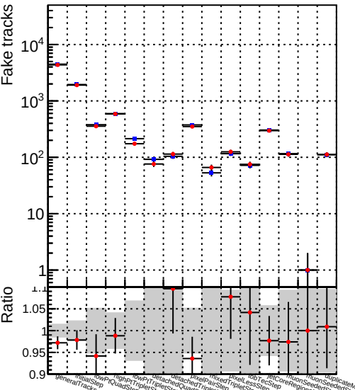
Numbe 1 DQM_CKF_XiMinusNOPU_retrainOldFiles125_v2_prelimWPM_epoch4
