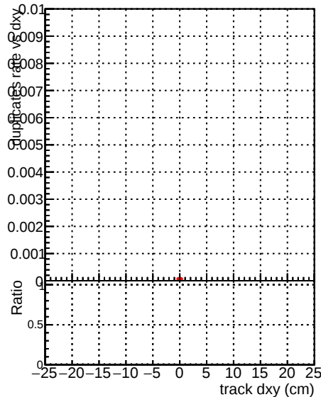
—●— DQM_CKF_XiMinusNOPU_base —●— DQM_CKF_XiMinusNOPU_retrainOldFiles125_v2_prelimWPM_epoch4
