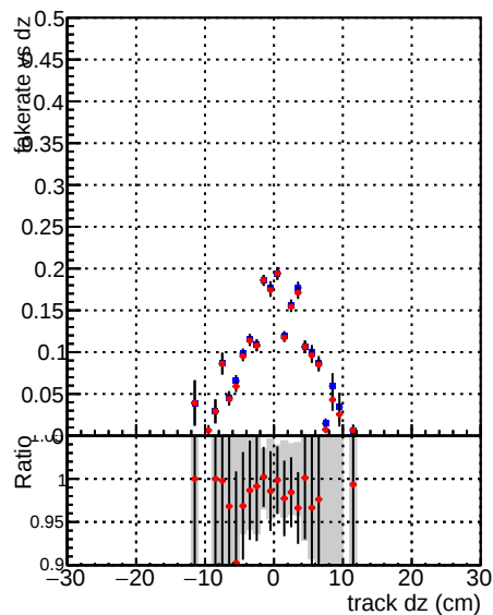
—●— DQM_CKF_XiMinusNOPU_base —●— DQM_CKF_XiMinusNOPU_retrainOldFiles125_v2_prelimWPM_epoch4
