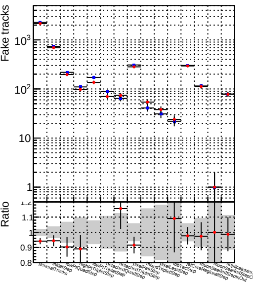
Numbe 1 DQM_CKF_XiMinusNOPU_retrainOldFiles125_v2_prelimWPM_epoch4
